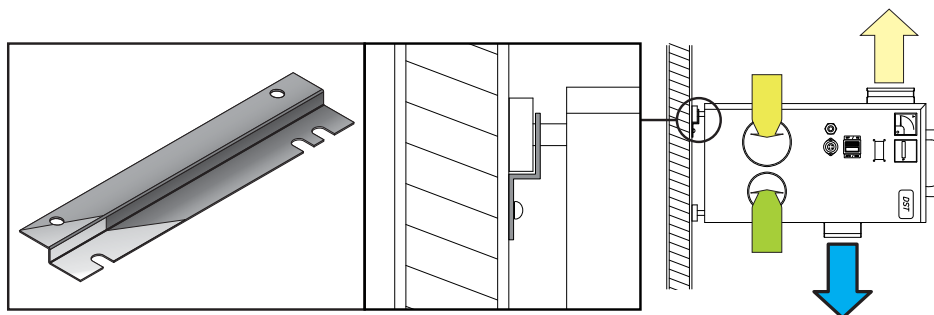
FIGURA 10: Soporte para montaje en pared
