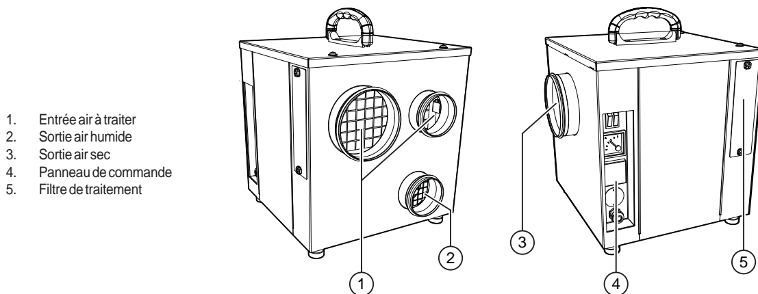
IMAGE 4: Vue d'ensemble du produit
