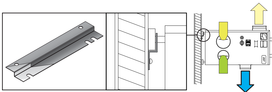
FIGUR 8: Stålfästen för väggmontering
