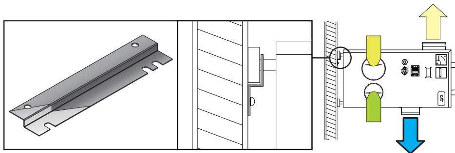
FIGUR 6: Stålfästen för väggmontering
