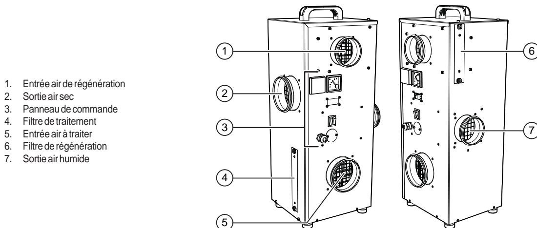
IMAGE 4: Vue d'ensemble du produit
