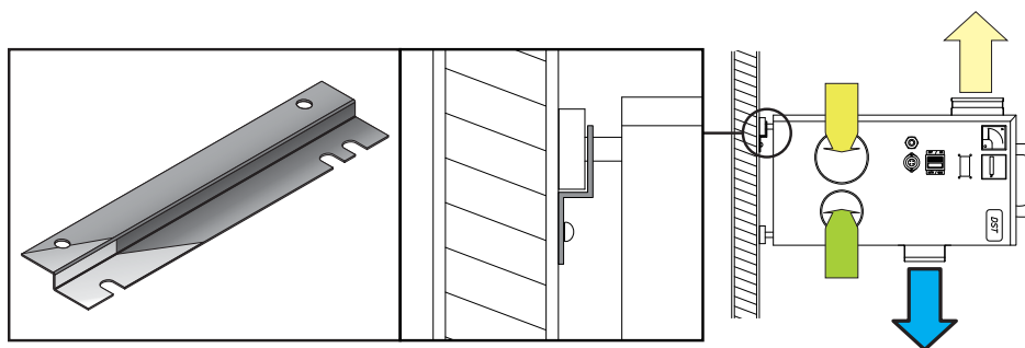
IMAGE 8: Support pour montage mural
