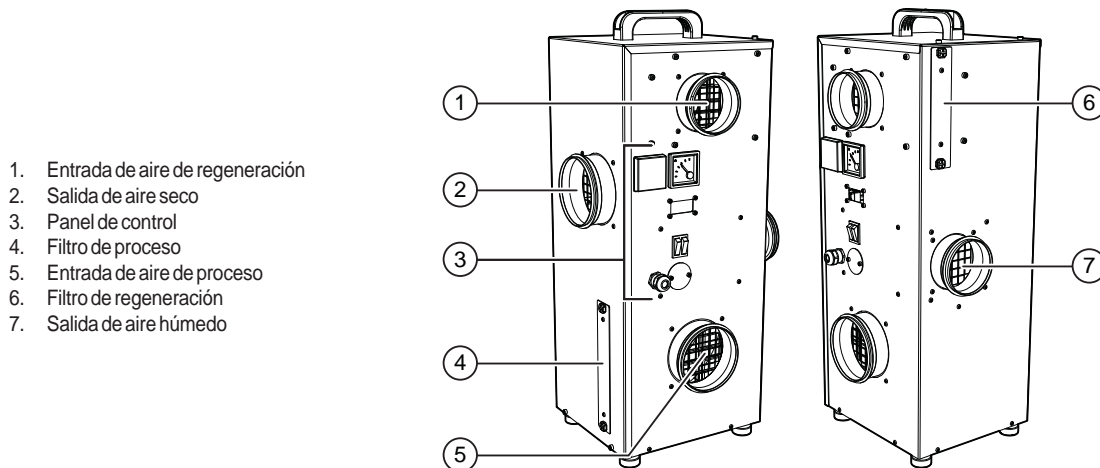
FIGURA4: Vista general del producto
